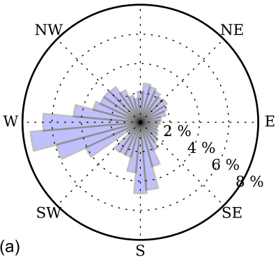
Alturas wind rose
